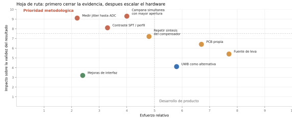
Figura 16: Hoja de ruta de validación, ordenada por dependencia y por valor de la evidencia que aporta cada ensayo pendiente.
