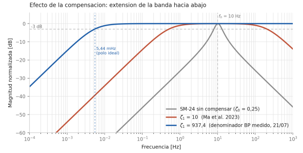
Figura 6: Efecto de la compensación sobre la respuesta referida a aceleración. Al elevar \zeta_1 los polos complejos se separan en dos reales, y el inferior desplaza el quiebre f_1 hacia la banda de interés.
