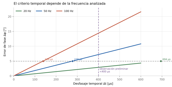
Figura 2: Traducción del desalineamiento temporal entre canales a error de fase y, a través de la geometría, a error de velocidad de fase. El presupuesto fija el criterio de medición de la sincronización.
