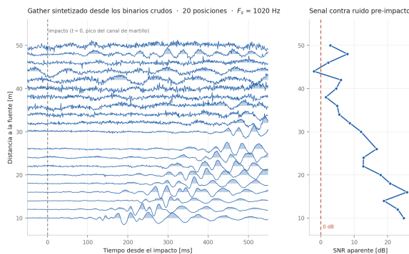
Figura 13: Registro multicanal sintetizado por posiciones, ensamblado desde los binarios crudos de la campaña, una traza por posición.
