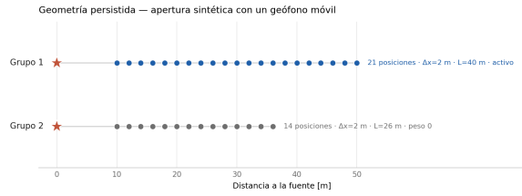
Figura 11: Geometría conservada en el estado de procesamiento: 21 posiciones con paso nominal de 2 m y apertura L = 40 m. El trazado es aproximado por no disponerse de relevamiento de coordenadas.
