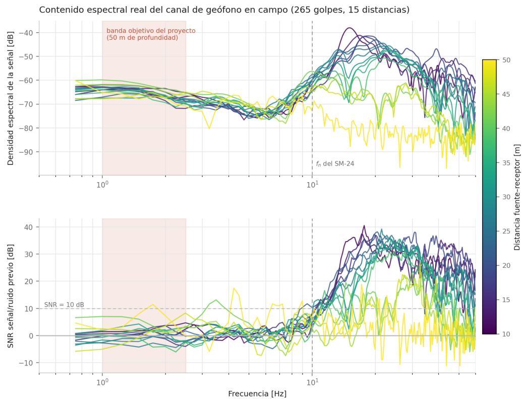
Figura 12: Arriba: densidad espectral de la señal por distancia. Abajo: relación señal a ruido contra el ruido previo al disparo. La banda sombreada es el objetivo de baja frecuencia que hoy no se alcanza.
