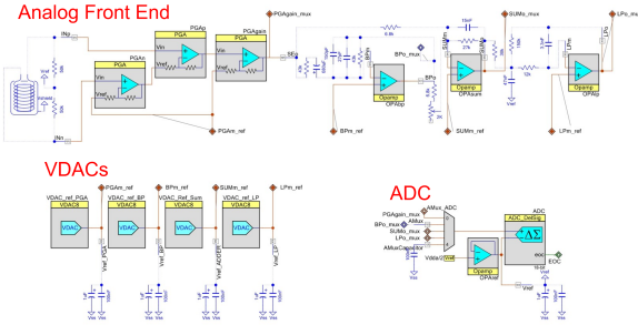
Figura 5: Cadena analógica implementada: entrada instrumental y ganancia programable, rama pasabanda de compensación, sumador y filtrado pasa-bajos previo al convertidor.
