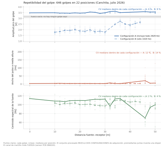
Figura 9: Repetibilidad del impacto medida sobre el canal del martillo. Los puntos claros son golpes individuales y las líneas la mediana por posición.
