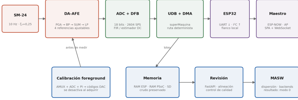
Figura 3: Arquitectura vigente del sistema y frontera entre el camino determinista de muestra y las funciones de calibración, comunicación y almacenamiento.
