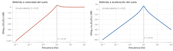
Figura 4: Respuesta nominal del SM-24 en circuito abierto, con las formas referidas a velocidad y a aceleración sobre los mismos ejes. Bajo f_n caen a razón de 40 y 20 dB por década respectivamente; son dos referencias de la misma tensión de salida, no dos modos de funcionamiento.
