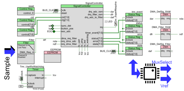
Figura 8: Camino digital implementado en el PSoC: convertidor, filtro FIR por hardware, canales DMA y bloque de control descrito en lógica programable.
