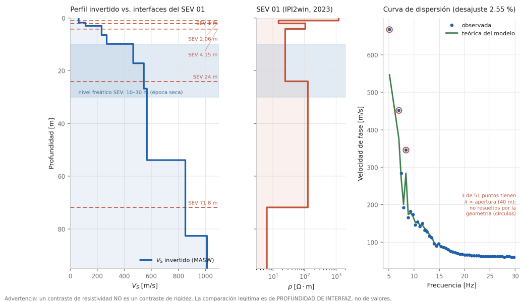
Figura 15: Contraste del perfil V_S invertido contra el modelo geoelectrico del SEV 01. Las técnicas miden propiedades distintas: la coincidencia debe leerse como compatibilidad en el intervalo de 2 a 4 m, no como acuerdo puntual.
